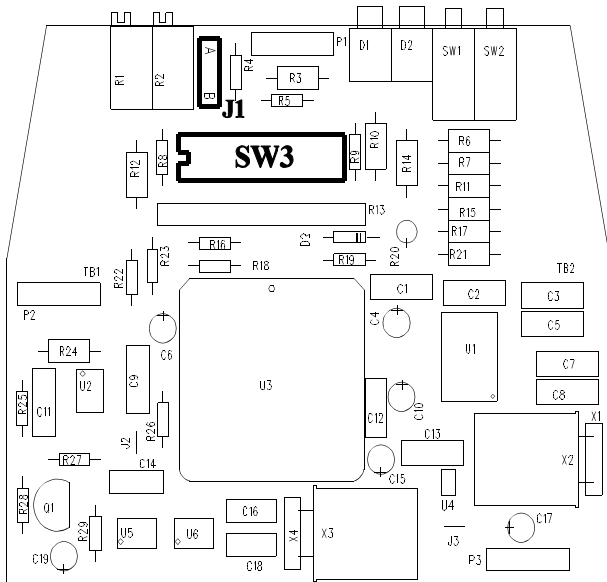
Input PCB
