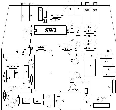
Input PCB
