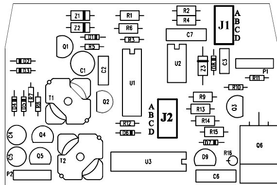
Output PCB
