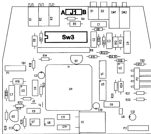
Input PCB
